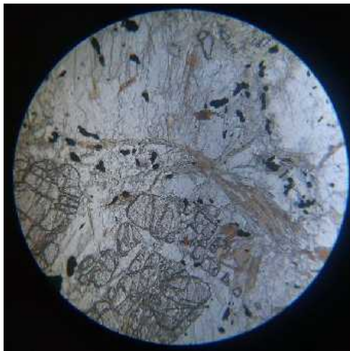
სურ. 6.8 კორდიერიტ – გრანატ – ბიოტიტ – პლაგიოკლასიანი ფელსი. ერთი ნიკოლი, X 64
