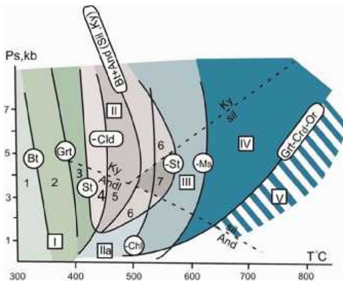
სურ 2.1. მეტამორფული ფაციესებისა და სუბფაციების გამარტივებული სქემა (Кориковский, 1979). რომელიც ციფრებით აღნიშნულია ფაციესები, არაბულით - სუბფაციები, მინერალების სიმბოლოებით კი - კრიტიკული მინერალების ან პარაგენეზისების გაჩენა და გაქრობა (-)
