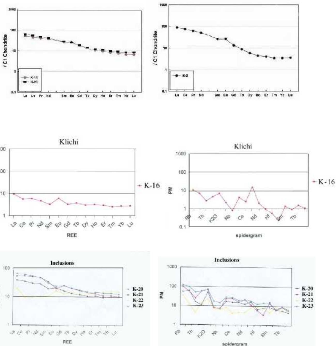
სურ 5.10 კლიჩის ინტრუზივის და სინმორფულ, ჰომოლოგიურ ავტოლითში იშვიათ და იშვიათმიწა ელემენტების განაწილების ამსახველი სპაიდერგრამები, სტანდარტიზებულია ქონდრიტზე (Taylor, McLennan, 1985).
