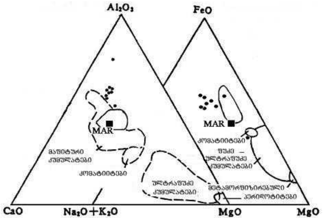
სურ. 5. 4. კლიჩის გაბრო-დიორიტული ორთოგნეისების ალმნიშვნელიფიკური წერტილების განლაგება ACM და AFM დიაგრამებზე (Колман, 1979).
